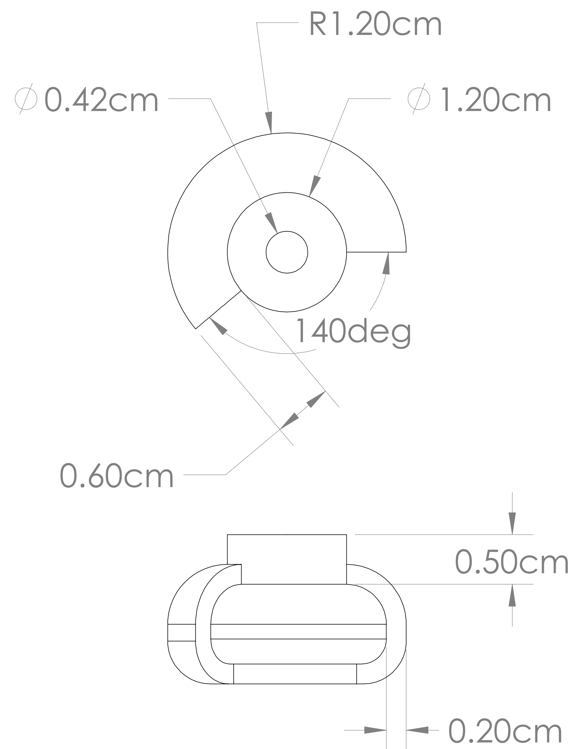
Pipette Plunger Cap
