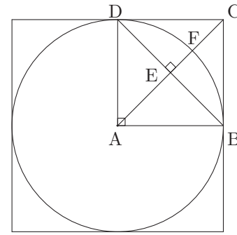
Fig. 48: Internal tangent circle
