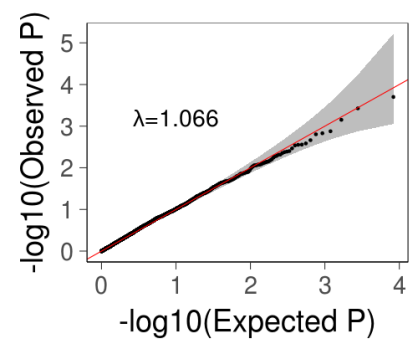
ORF
